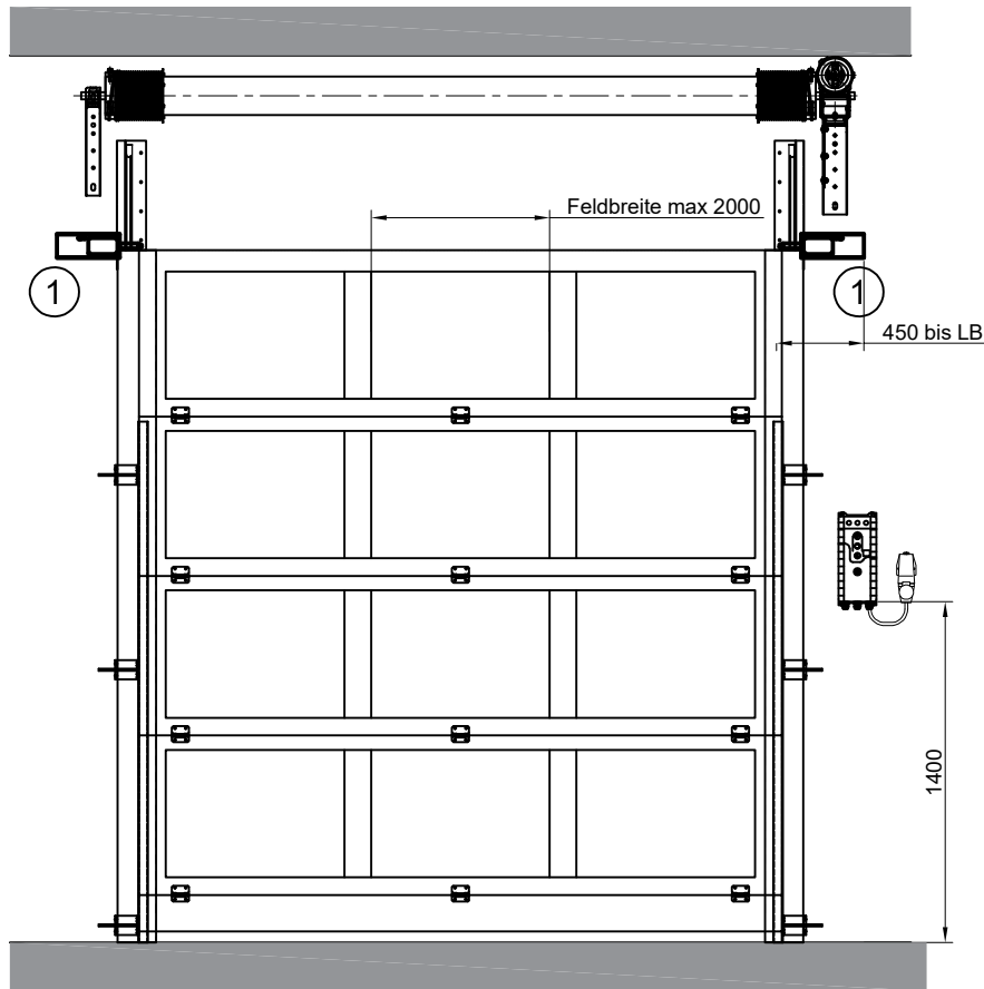
Gesamtansicht Innen
