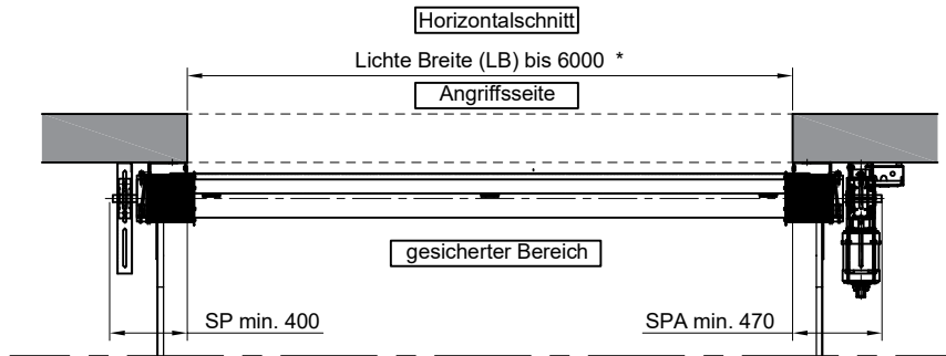
Horizontalschnitt
