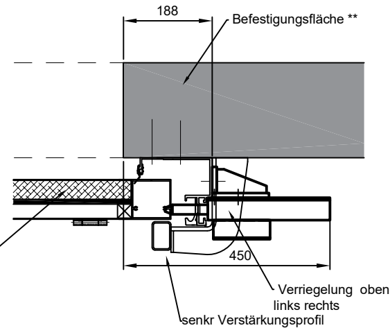
Detail Laufschiene Horizontalschnitt
