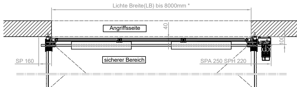
Horizontalschnitt
