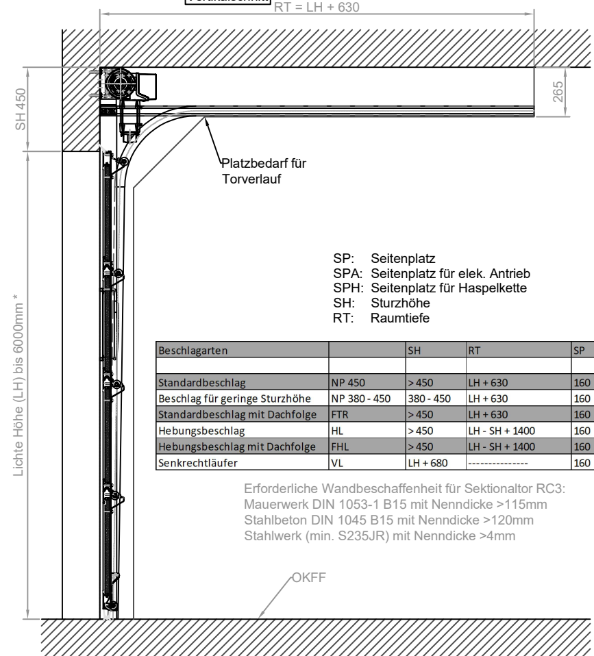
Vertikalschnitt
